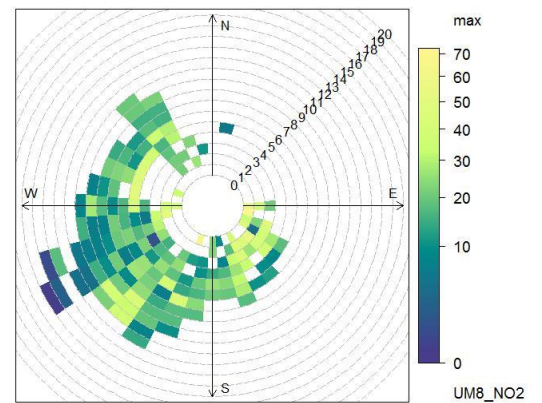
Rose de pollution [Lumbres_Hiver2016] - UM8_NO2 Concentrations maximales en fonction de la vitesse et de la direction du vent de Sangatte
