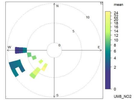
Rose de pollution - UM8_NO2 Concentrations moyennes en fonction de la vitesse et de la direction du vent de Sangatte [31/01/2016]
