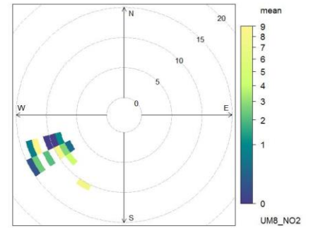
Rose de pollution - UM8_NO2 Concentrations moyennes en fonction de la vitesse et de la direction du vent de Sangatte [08/02/2016]
